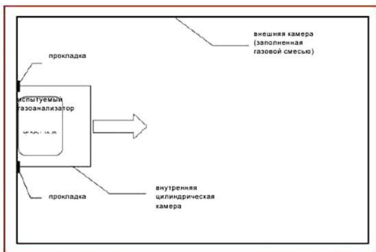
Рисунок В.5 - Пример применения метода вставки
