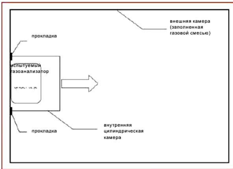
Рисунок В.3 - Пример применения испытательной камеры (вариант 2)
