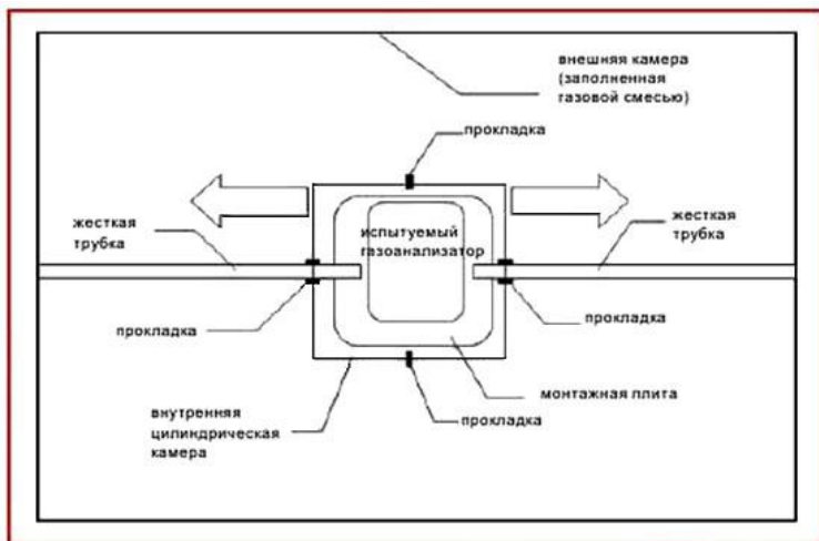
Рисунок В.2 - Пример применения испытательной камеры (вариант 1)
