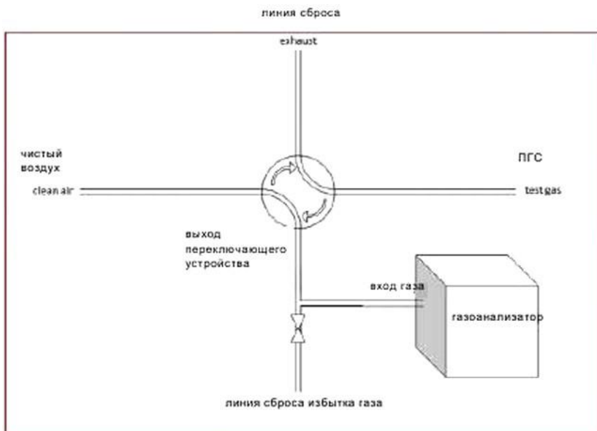
Рисунок В.1 - Схематическое изображение испытательной установки
