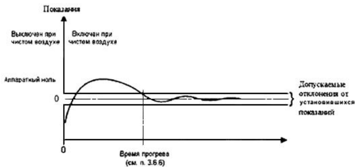
Рисунок 1 - Время прогрева в чистом воздухе
