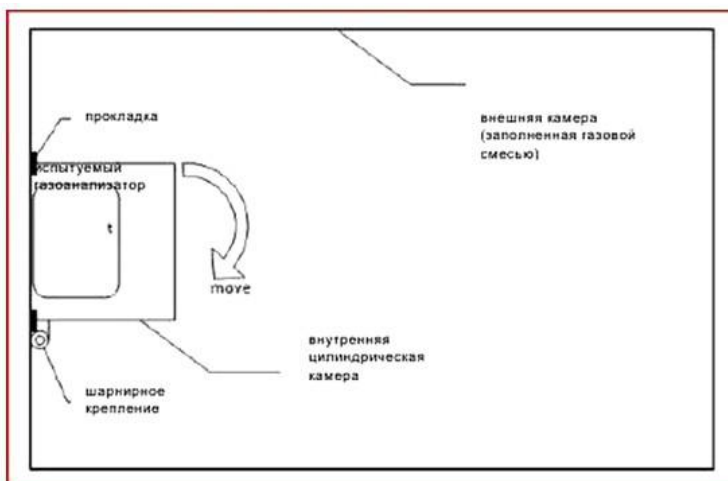
Рисунок В.4 - Пример применения испытательной камеры (вариант 5)
