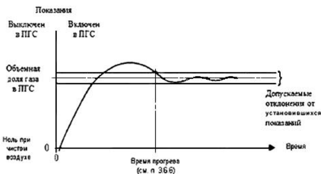
Рисунок 2 - Время прогрева в ПГС
